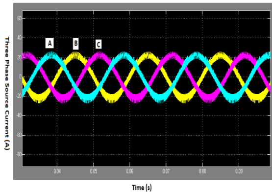
(b) ). Source current
