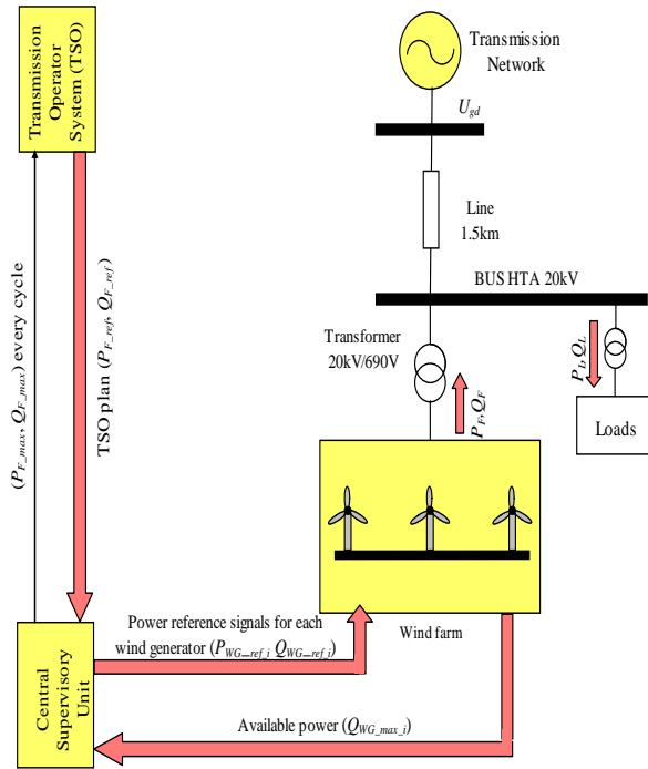
Fig.1 Power System Configuration [28]
