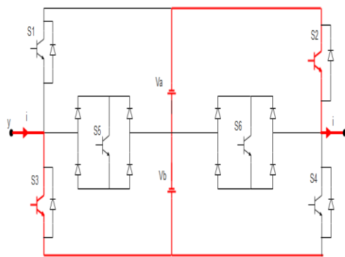
Mode 5: State 5 V_{xy} = + (V_1 + V_2) , S_2=S_3=1 ,
